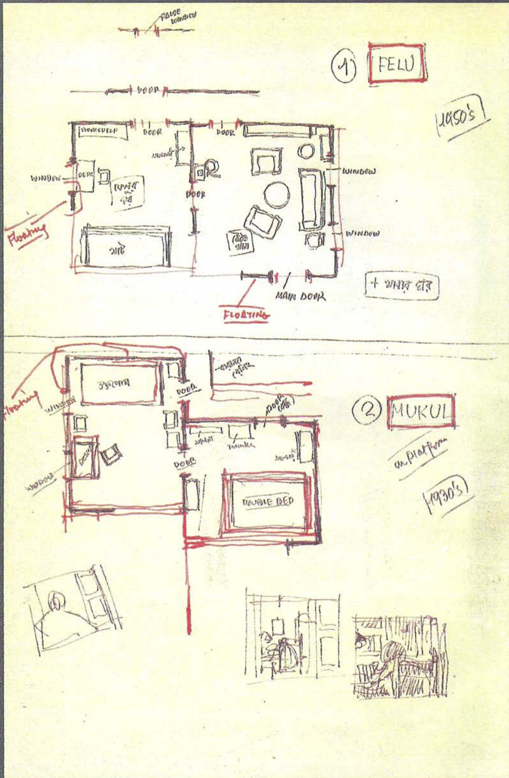
ইন্দ্রপুরী স্টুডিওতে তৈরি ফেলুদা ও মুকুলের বাড়ির ফ্লোর-প্ল্যান।
